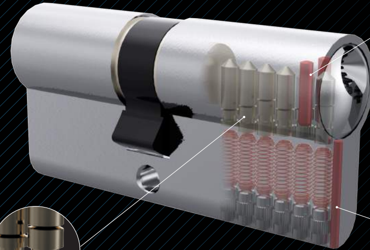
Aufbohrschutz (optional)
